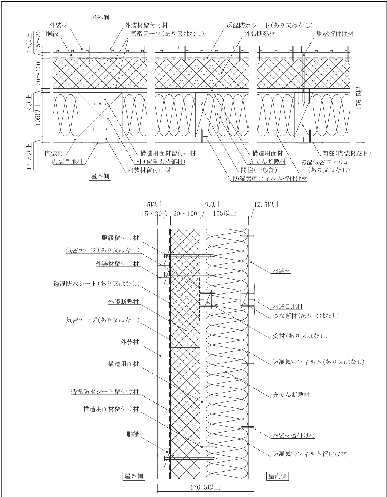
図4 構造説明図
