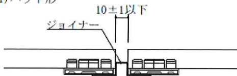
④金属ジョイナー目地
