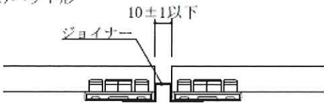
④金属ジョイナー目地 1)ハット形
